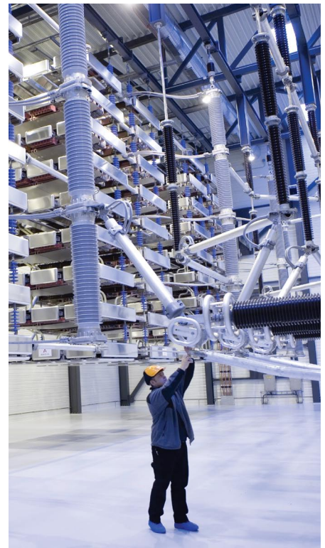
Tiristora ventilis ir Tjeles HVDC apakšstacijas, kas savieno Dāniju ar Norvēģiju, sirds. Te maiņstrāva tiek pārvērsta par līdzstrāvu un otrādi.
